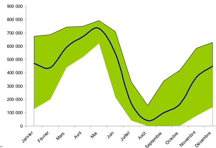
Profil de production - centrale "d'hiver"
